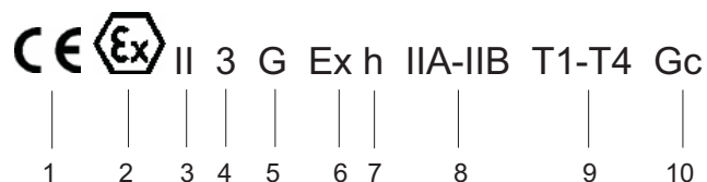
Abb. 16 Explosionsschutz-Kennzeichnung an der Pumpe (Gerätegruppe II, Kategorie 3)
