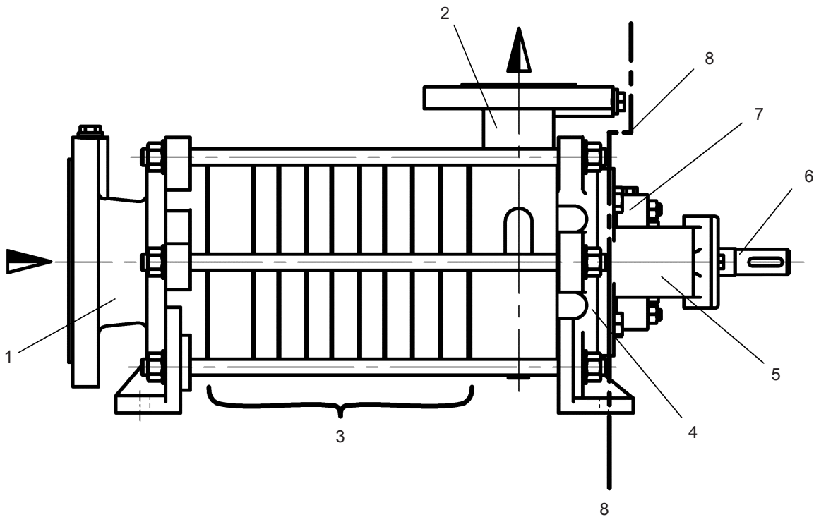
Abb. 4 Aufbau (Beispiel)
