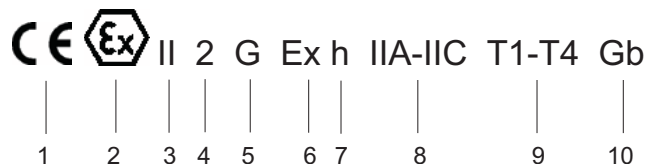
Abb. 15 Explosionsschutz-Kennzeichnung an der Pumpe (Gerätegruppe II, Kategorie 2)
