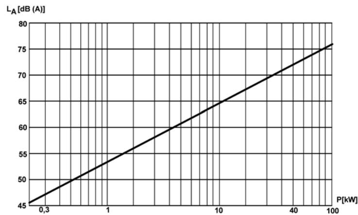
Abb. 14 Schalldruckpegel
