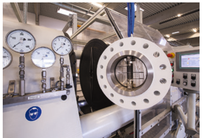
■ RITAG Rückschlagarmatur vom Typ ZRD vor der Prüfung RITAG check valve, type ZRD, before testing
